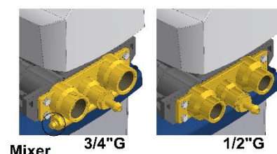
Attacchi idrici
